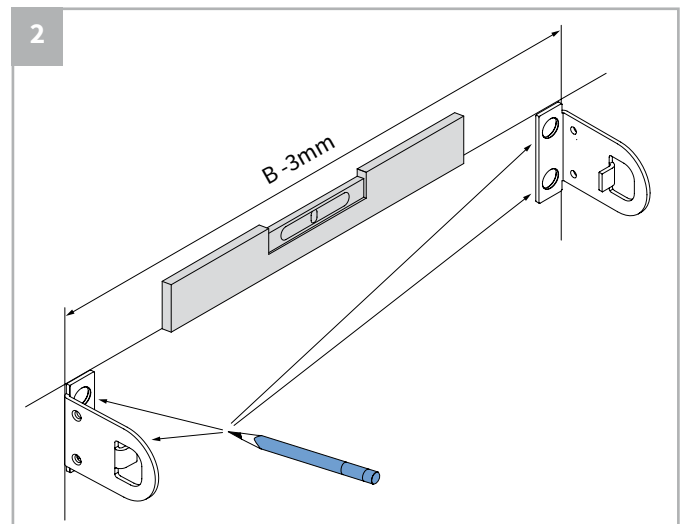
Plafondmontage
